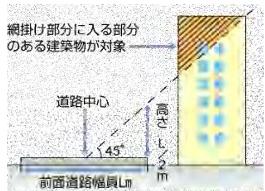
■図7 - 2 条例の基準となる建物のイメージ
